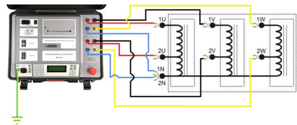
Conexión de TRT03 a autotransformador trifásico
