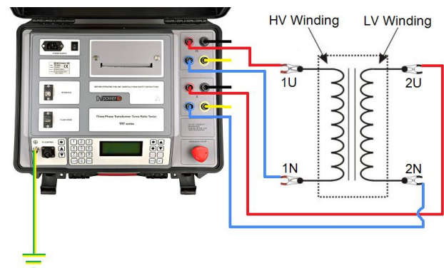
Conexión de TRT03 a transformador monofásico
