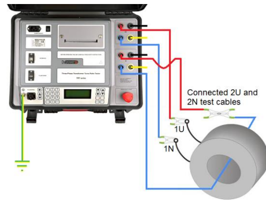
Conexión de TRT03 a un transformador de corriente amontado
