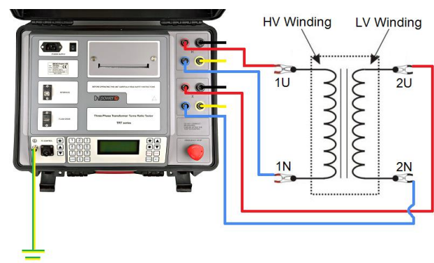
Conexión de TRT3x a transformador monofásico
