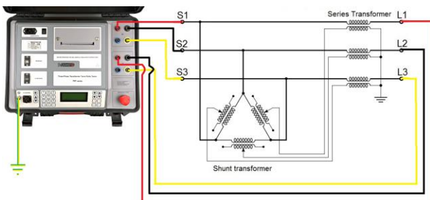
Conexión de TRT3x a transformador desfasador
