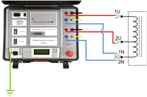
Conexión de TRT3x a autotransformador monofásico
