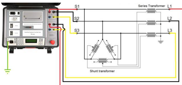
Conexión de TRT4x a transformador desfasador
