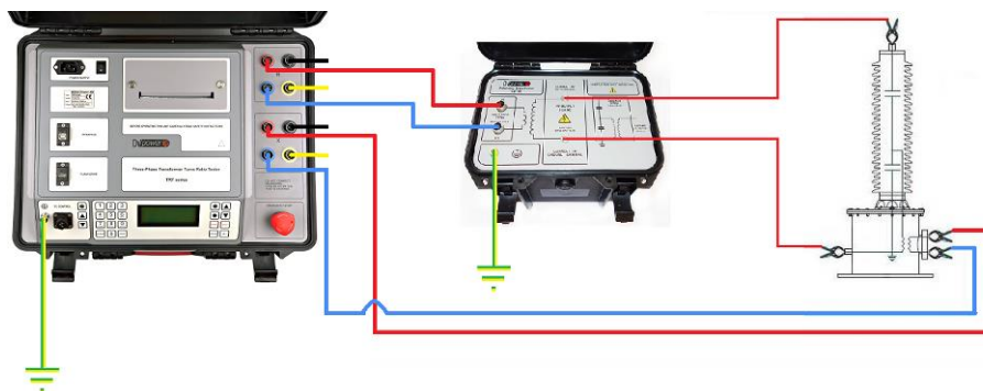
Conexión de TRT4x a transformador potencial capacitivo a través CVT40
