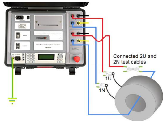
Conexión de TRT4x a un transformador de corriente amontado
